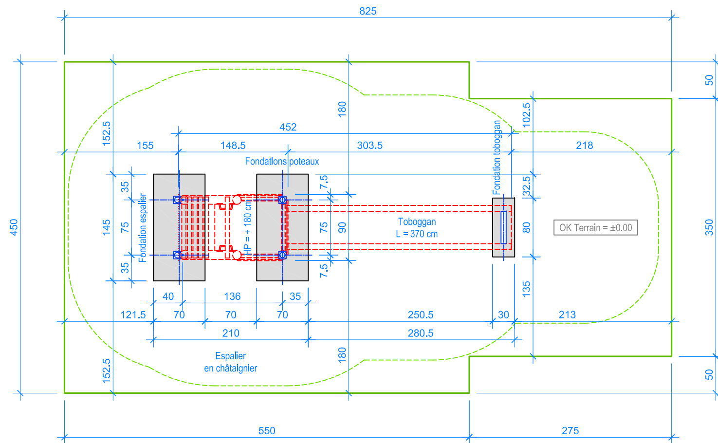
PLAN 1:50
