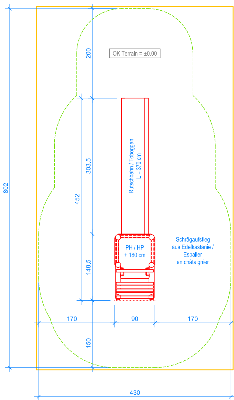
GRUNDRISS / PLAN 1:50
