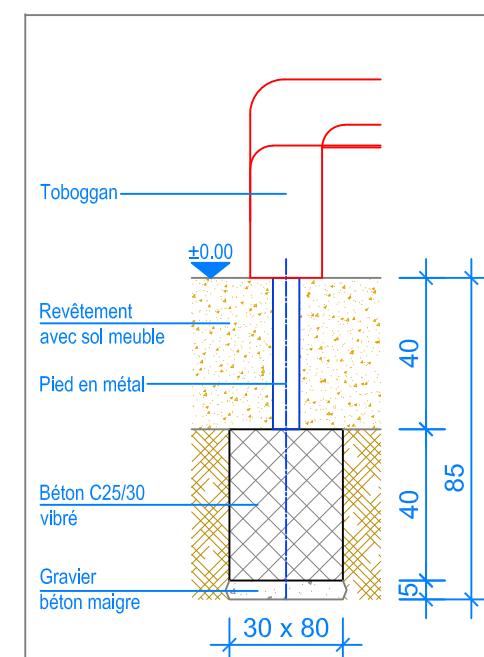
COUPE 1:20 FONDATION TOBOGGAN
