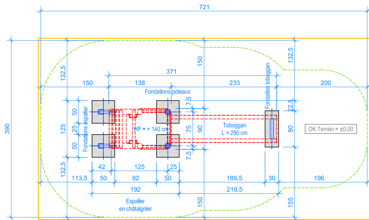
PLAN 1:50
