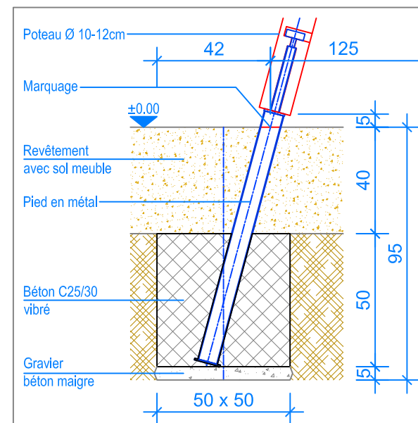
COUPE 1:20 FONDATION ESPALIER
