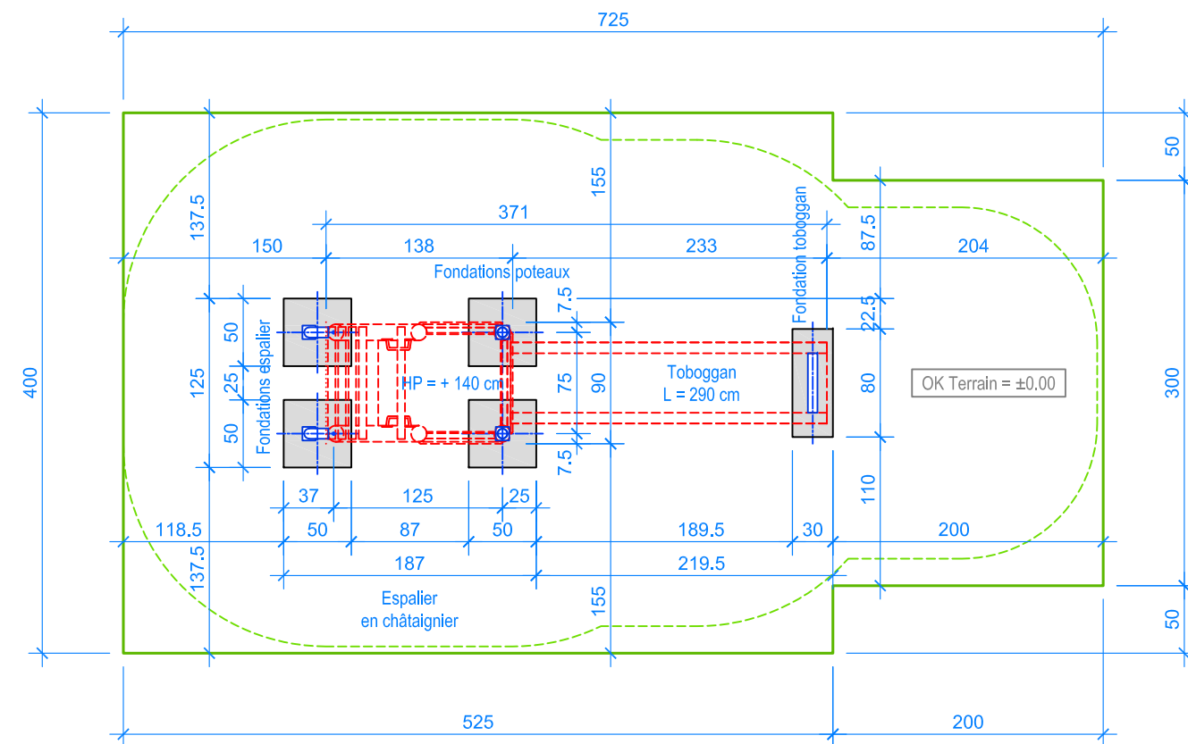
PLAN 1:50
