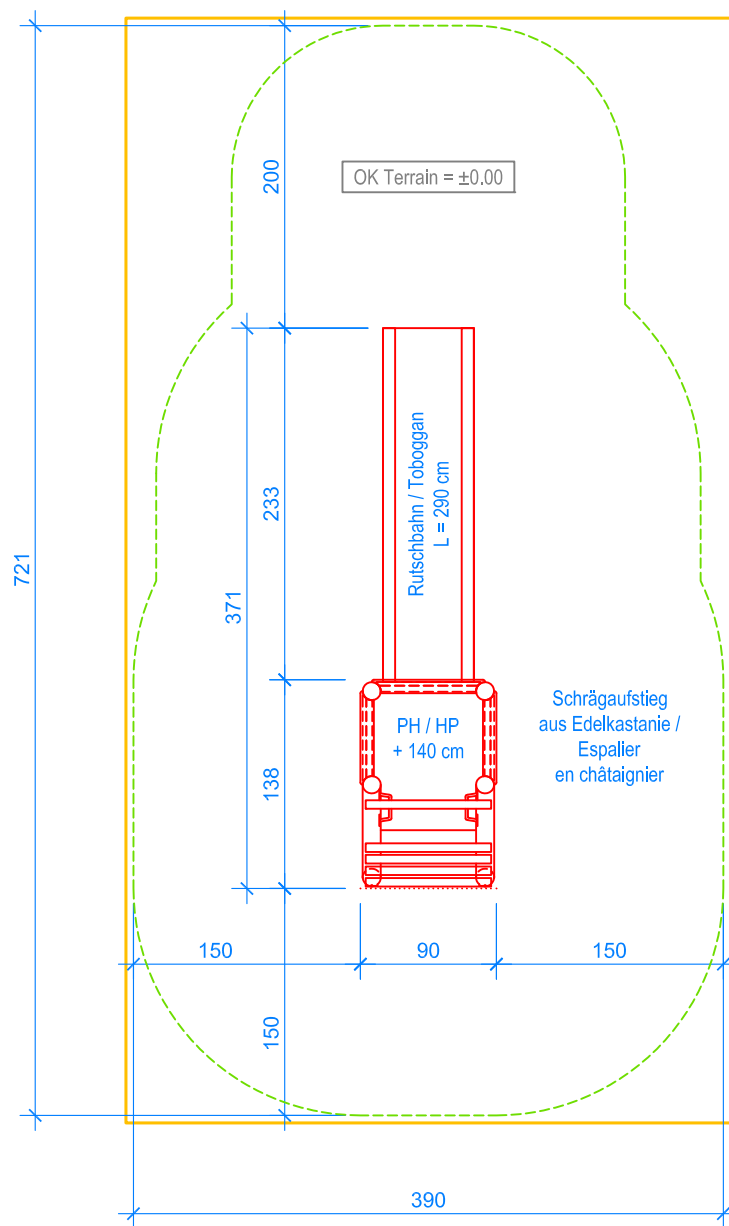
GRUNDRISS / PLAN 1:50
