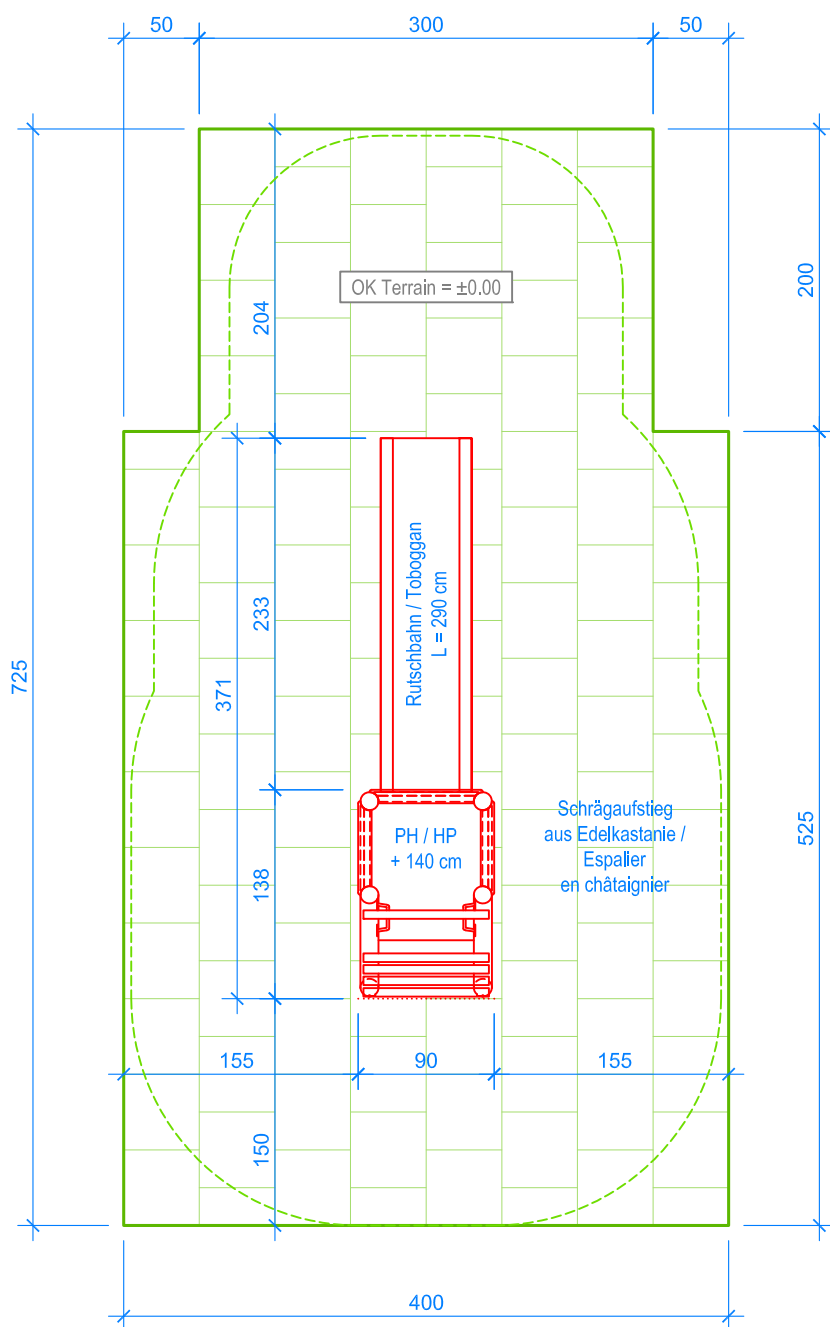
GRUNDRISS / PLAN 1:50
