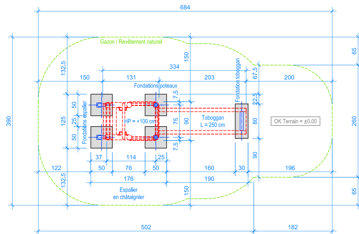
PLAN 1:50
