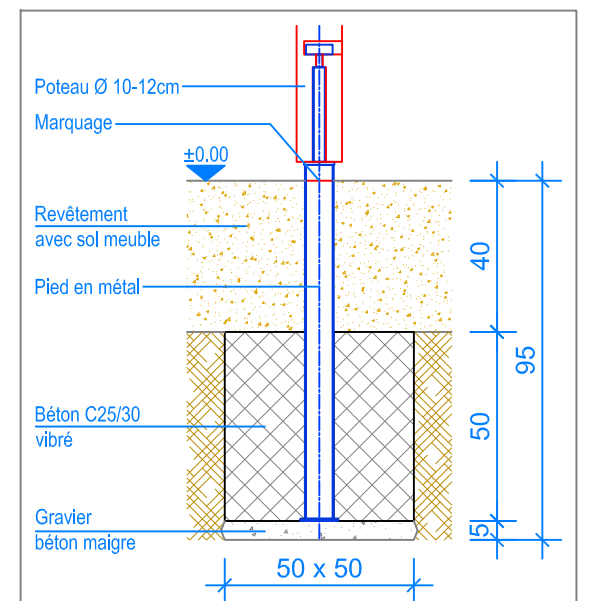
COUPE 1:20 FONDATION POTEAU
