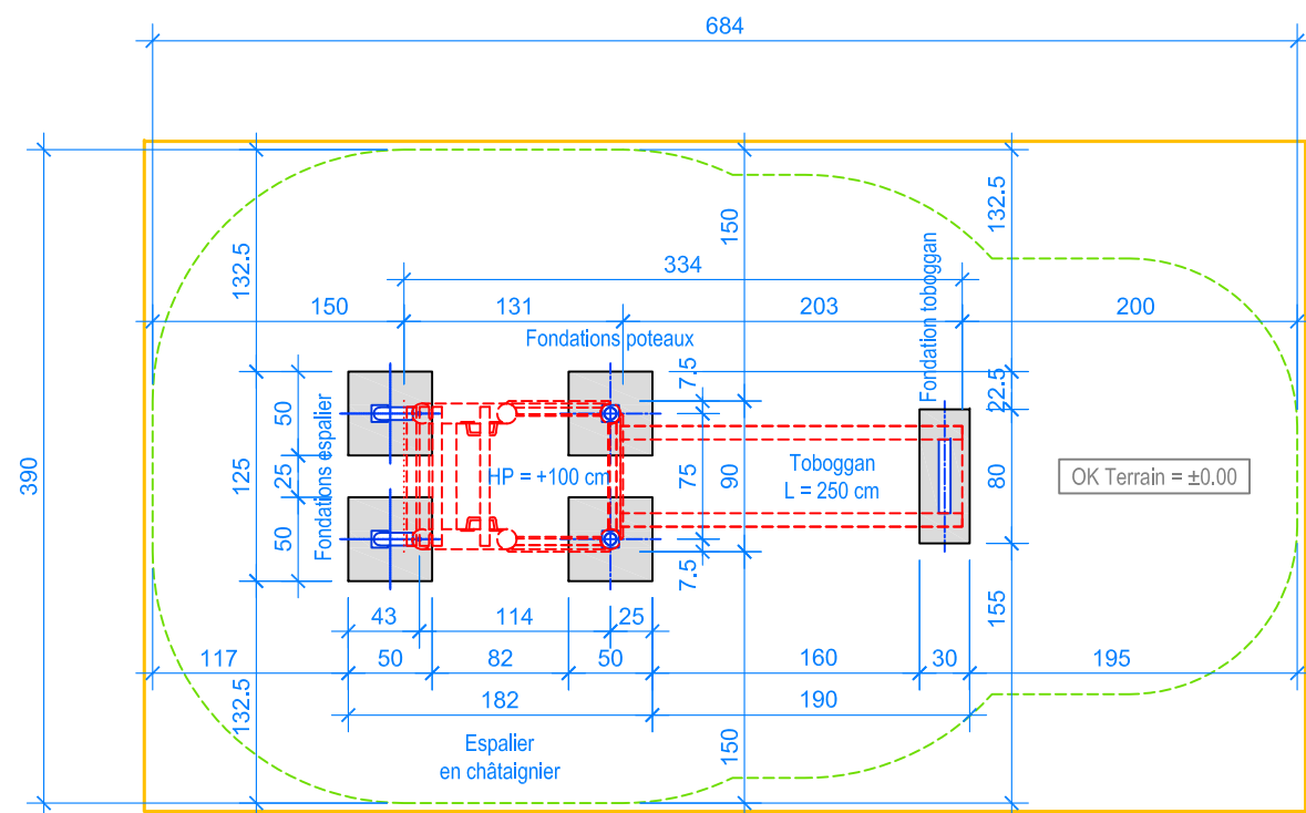
PLAN 1:50
