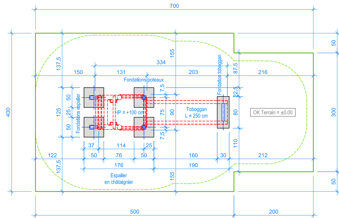
PLAN 1:50
