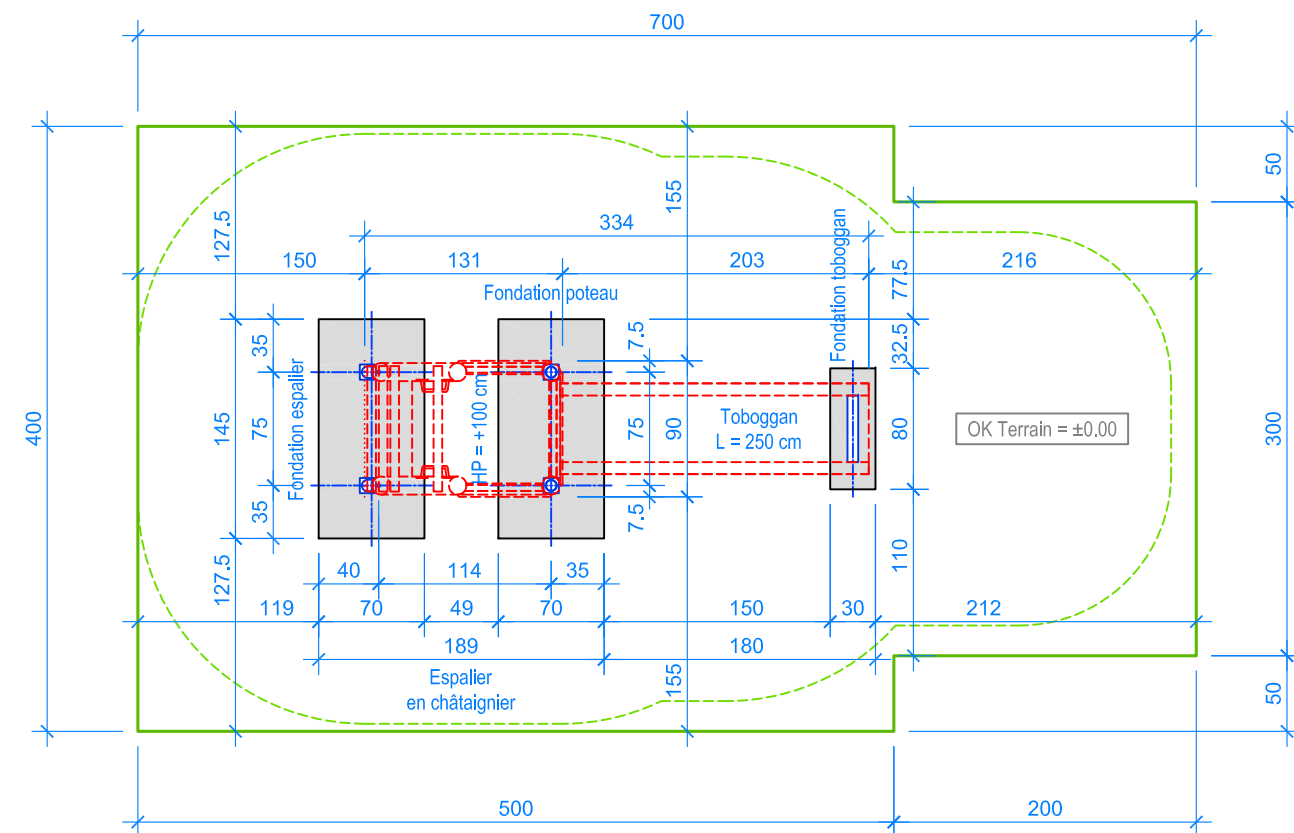
PLAN 1:50
