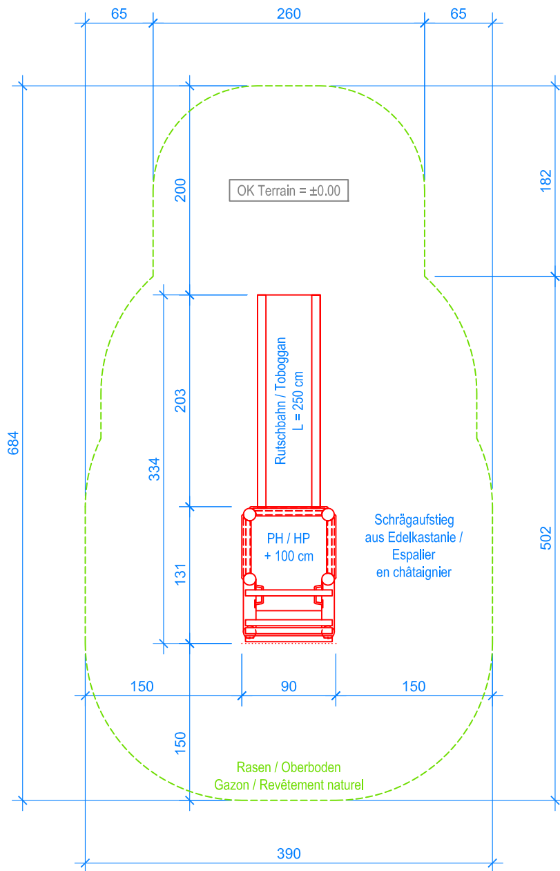
GRUNDRISS / PLAN 1:50
