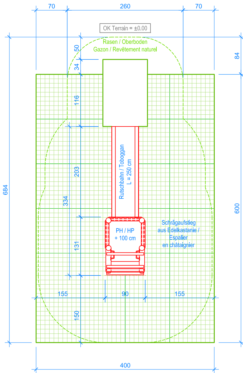
GRUNDRISS / PLAN 1:50
