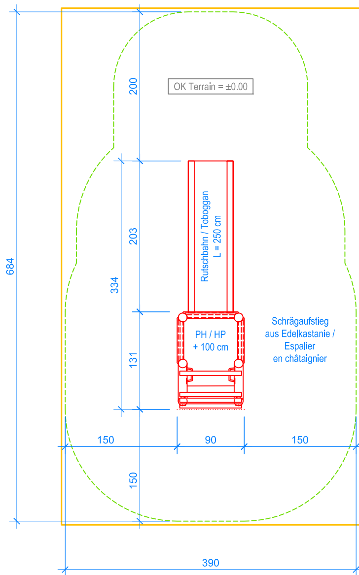
GRUNDRISS / PLAN 1:50
