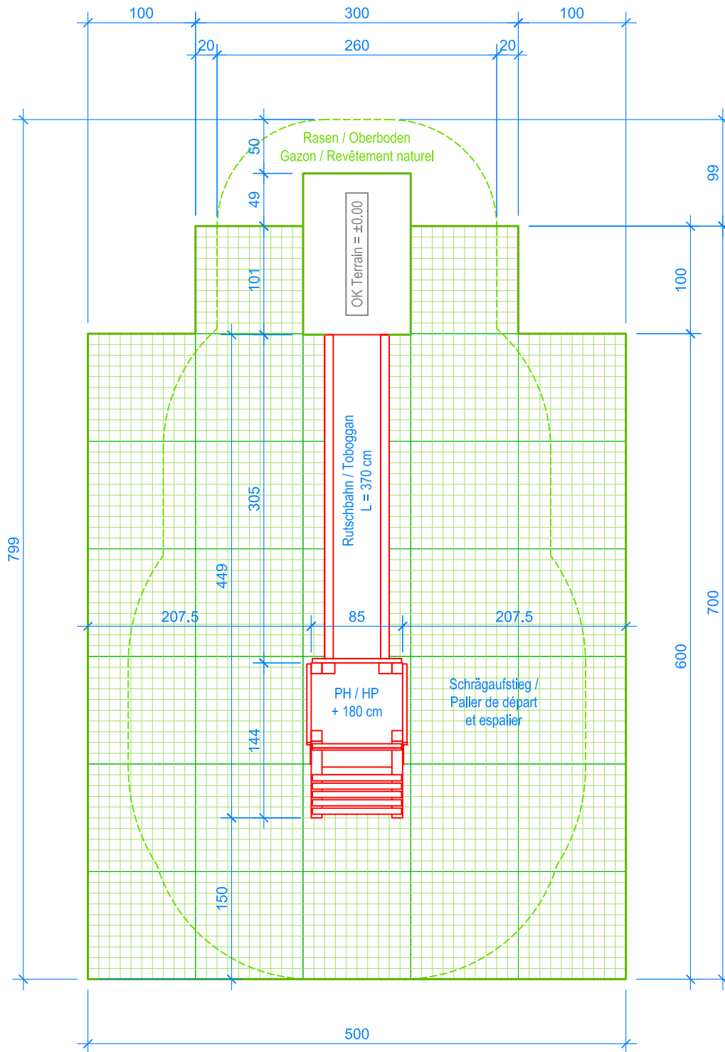
GRUNDRISS / PLAN 1:50
