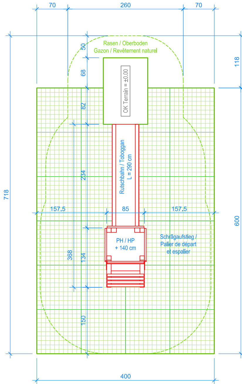
GRUNDRISS / PLAN 1:50
