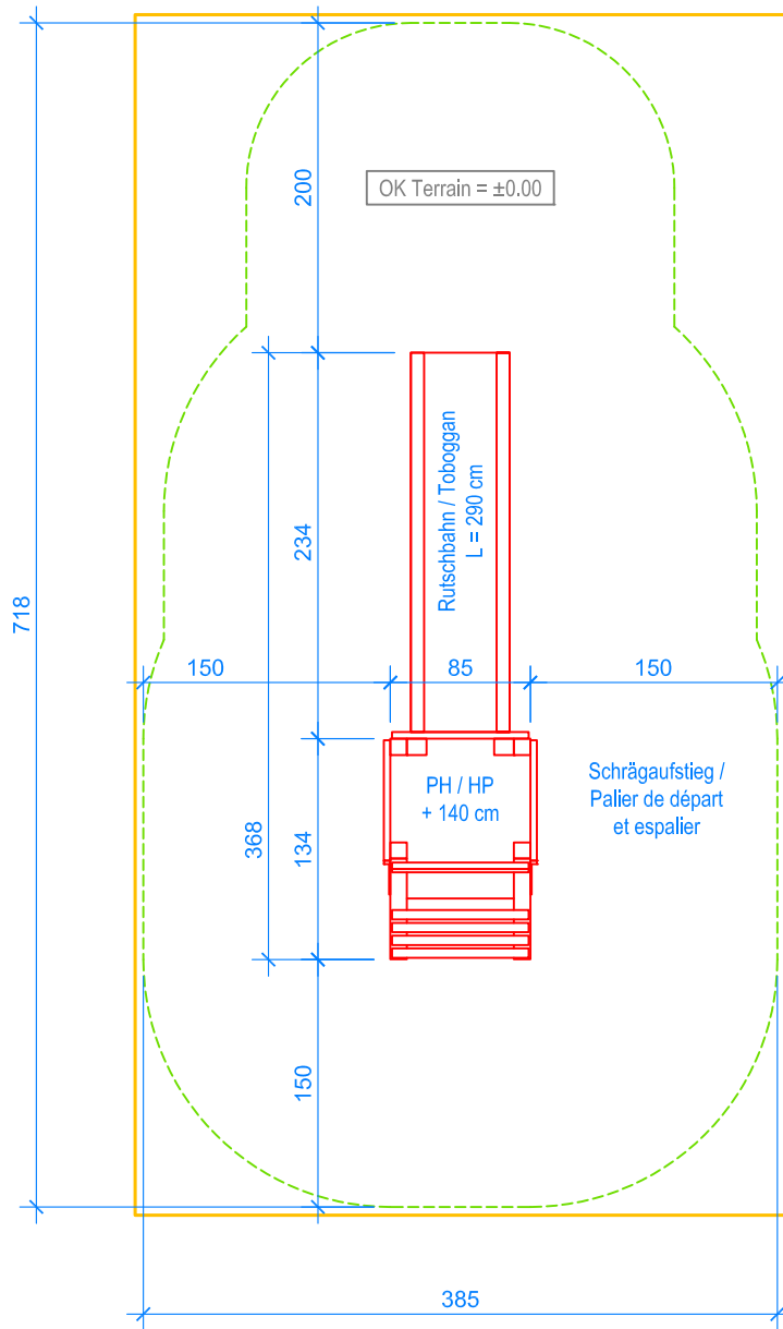
GRUNDRISS / PLAN 1:50
