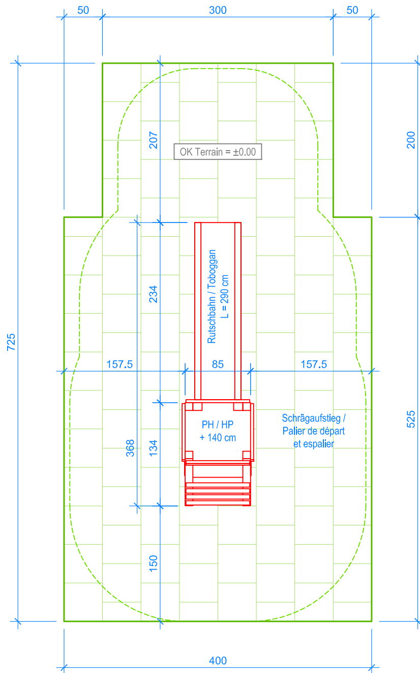
GRUNDRISS / PLAN 1:50
