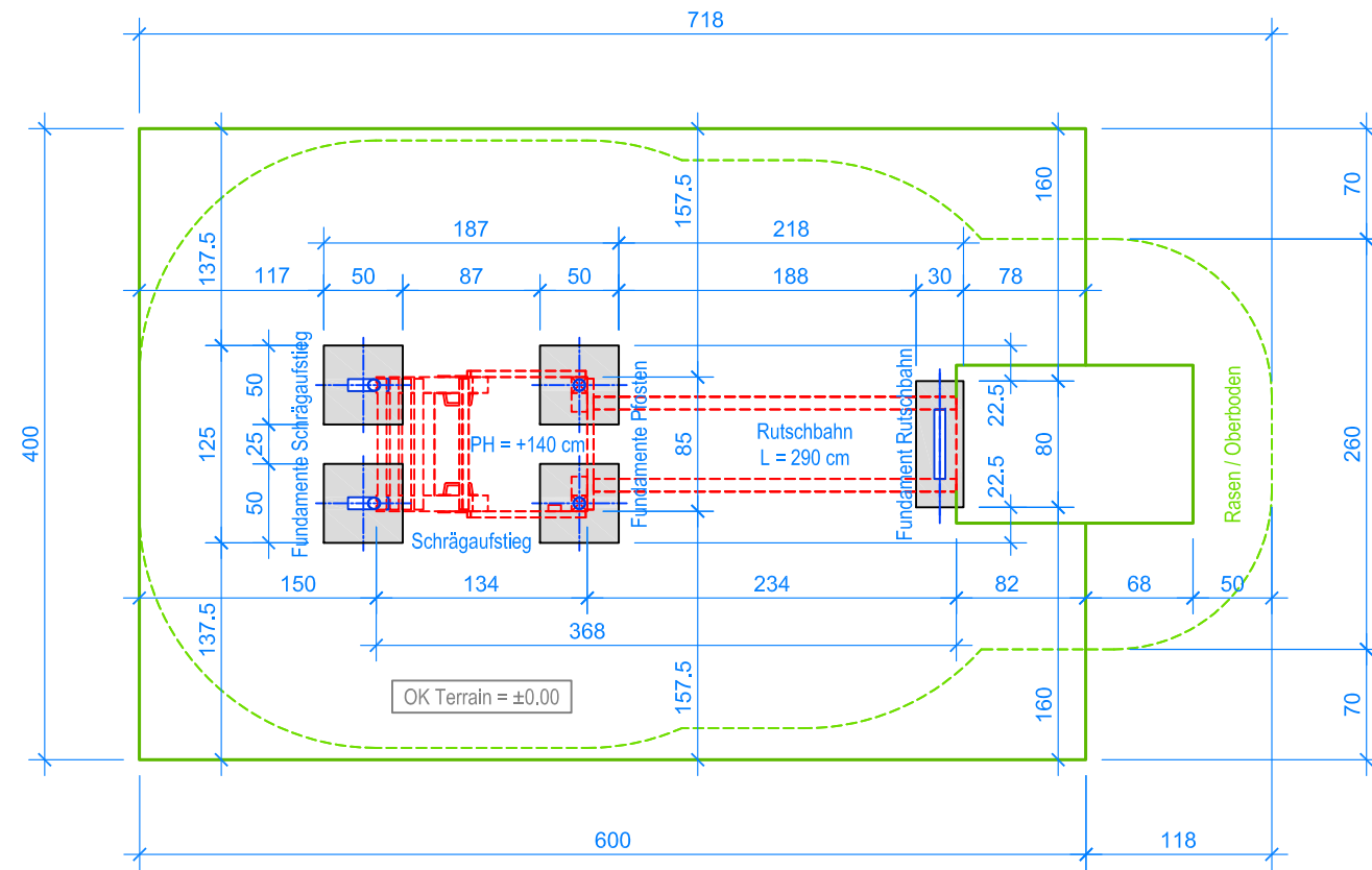
GRUNDRISS 1:50
