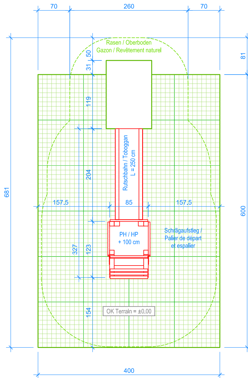
GRUNDRISS / PLAN 1:50
