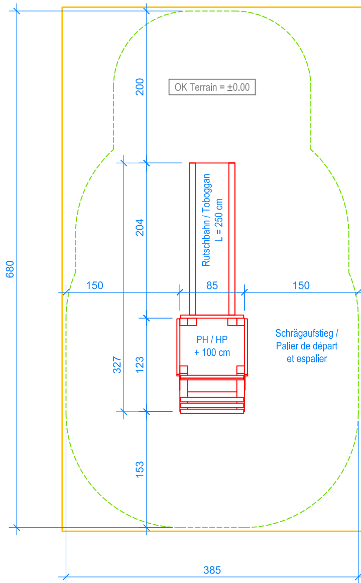
GRUNDRISS / PLAN 1:50
