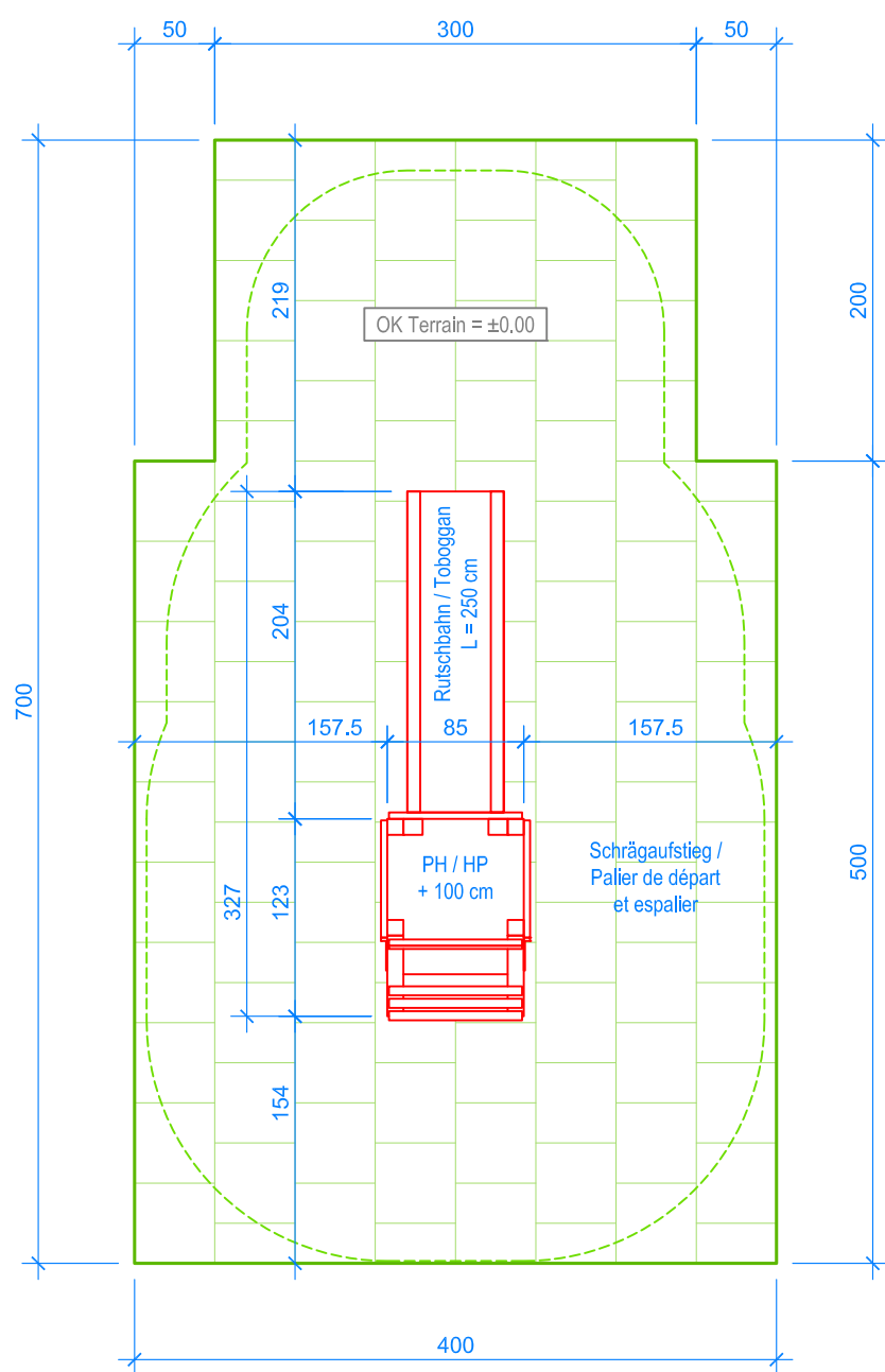
GRUNDRISS / PLAN 1:50
