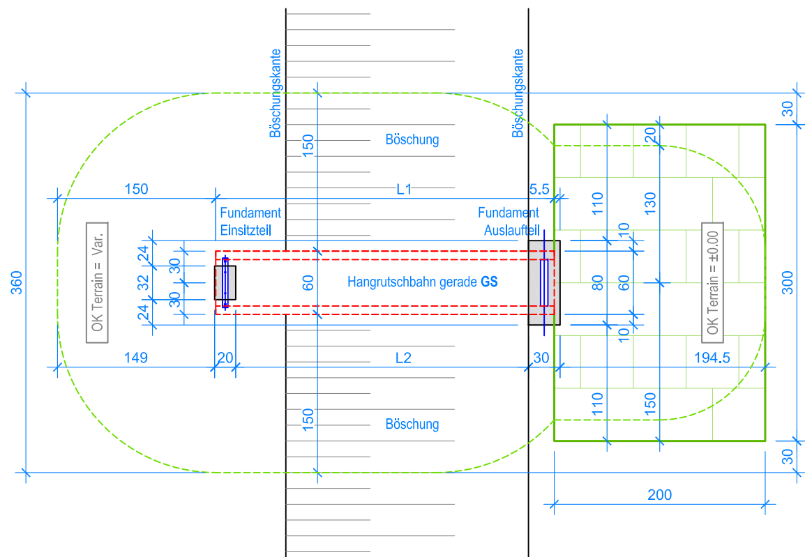
GRUNDRISS 1:50
