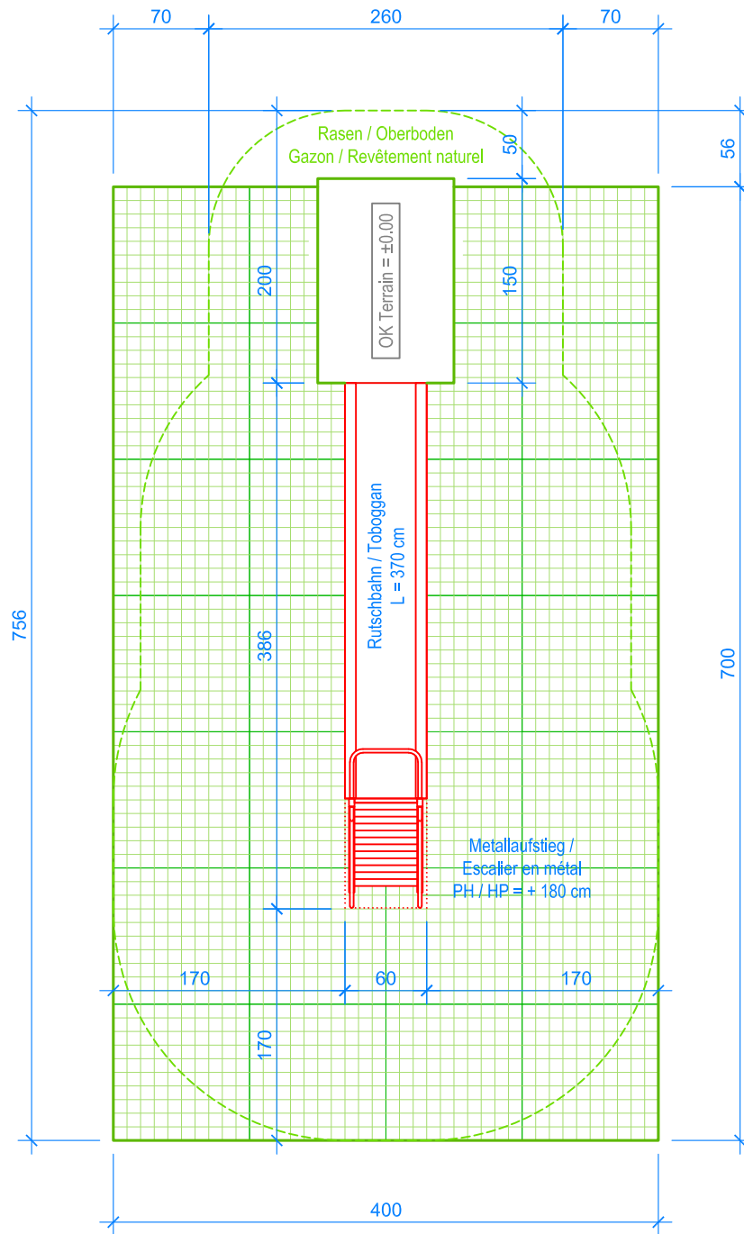
GRUNDRISS / PLAN 1:50
