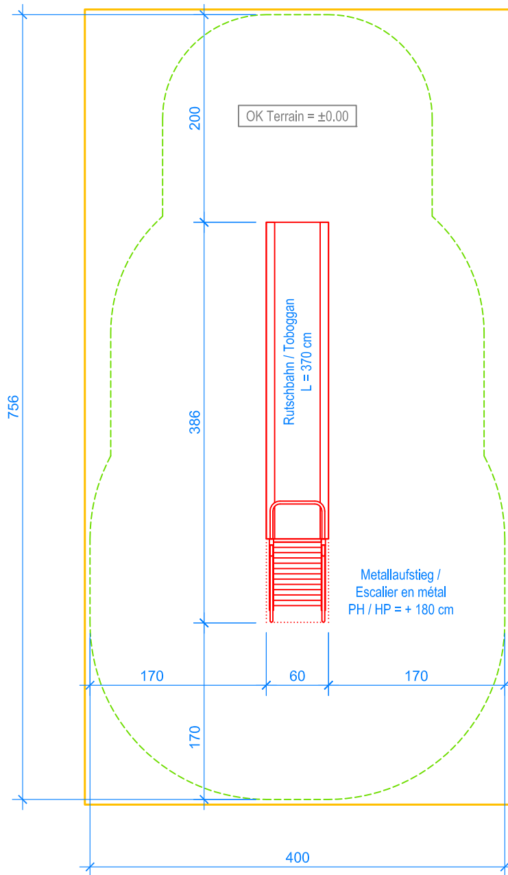
GRUNDRISS / PLAN 1:50
