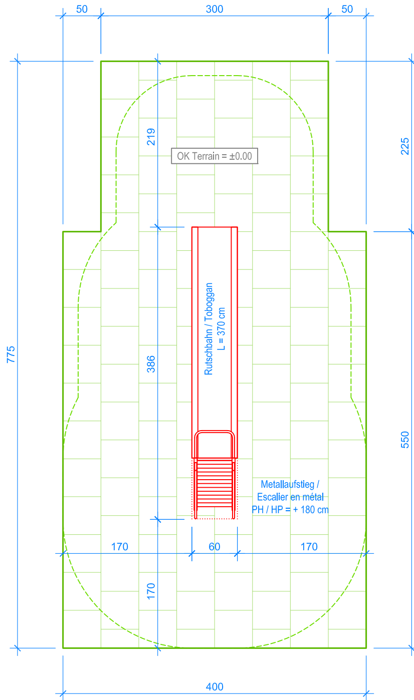
GRUNDRISS / PLAN 1:50
