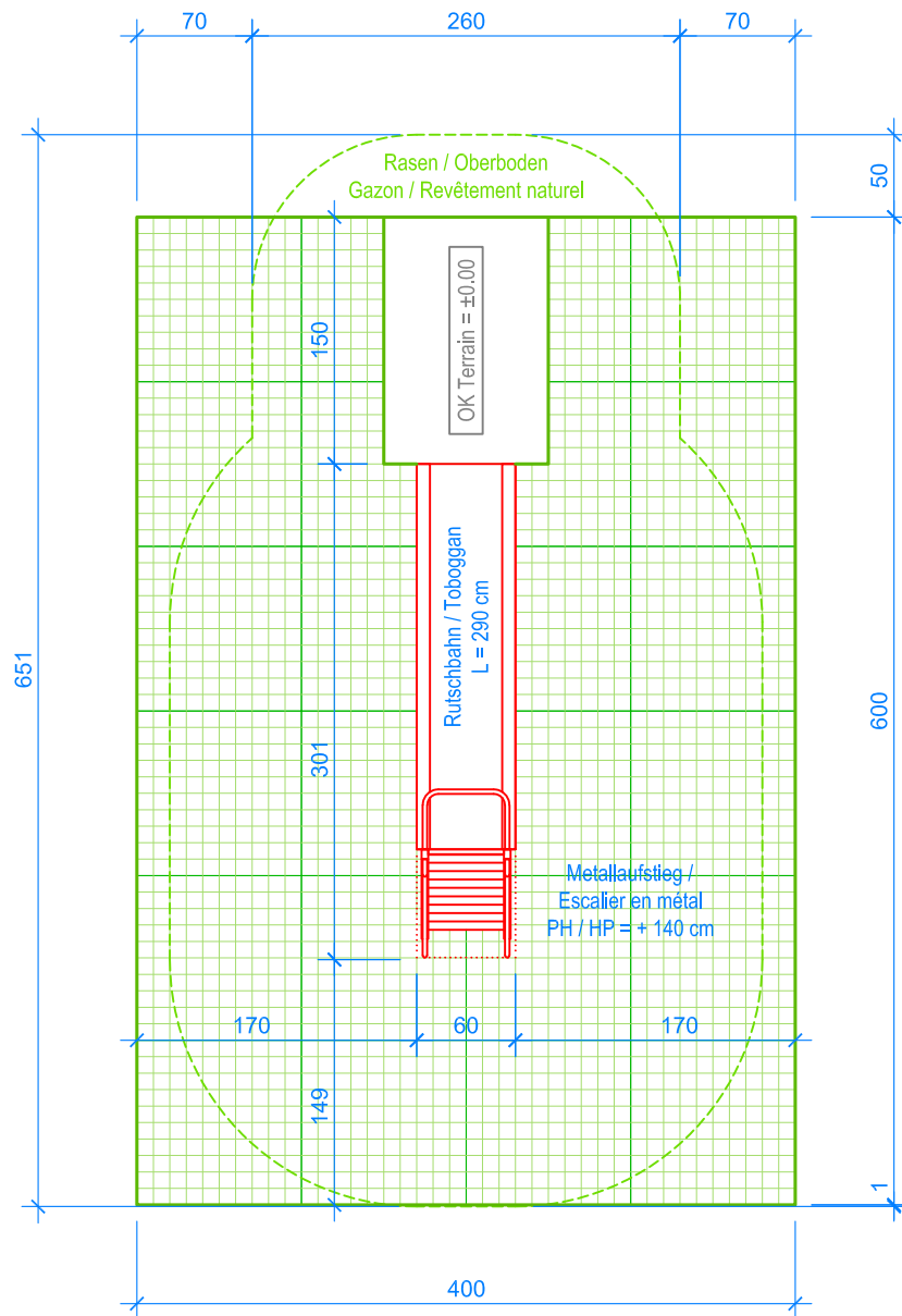
GRUNDRISS / PLAN 1:50
