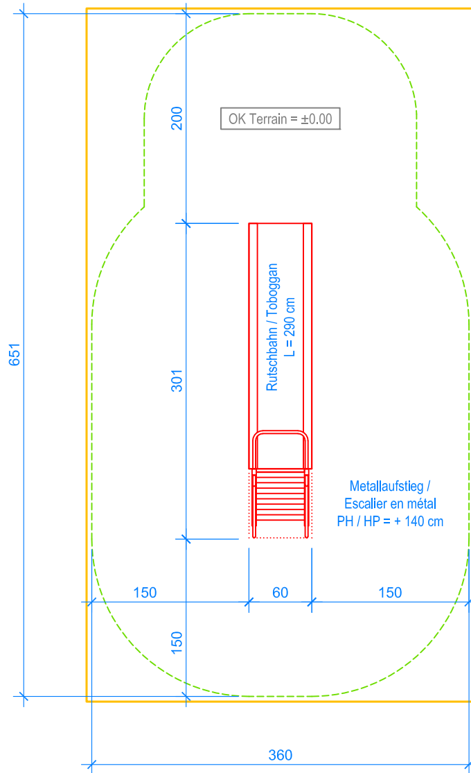
GRUNDRISS / PLAN 1:50
