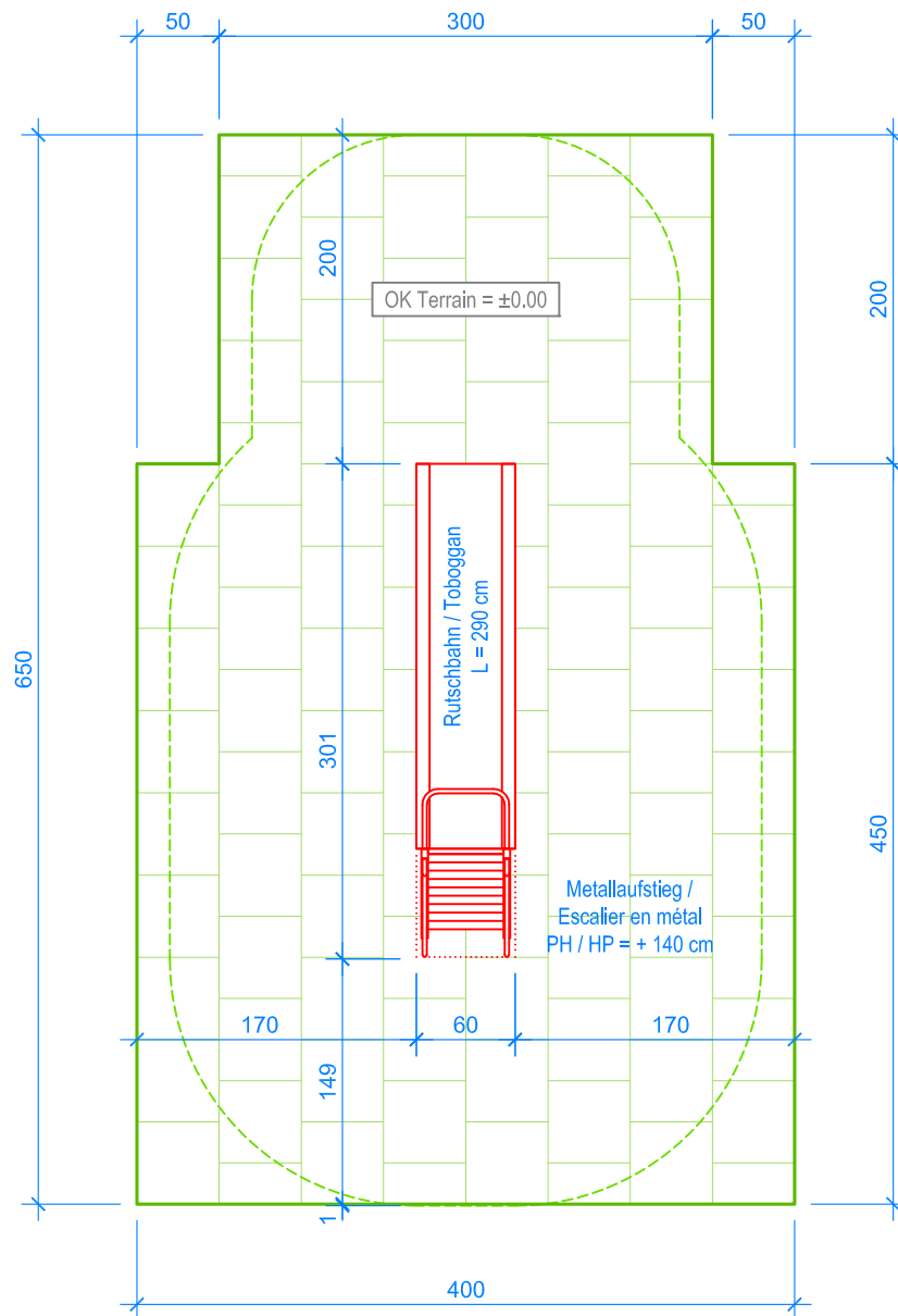
GRUNDRISS / PLAN 1:50
