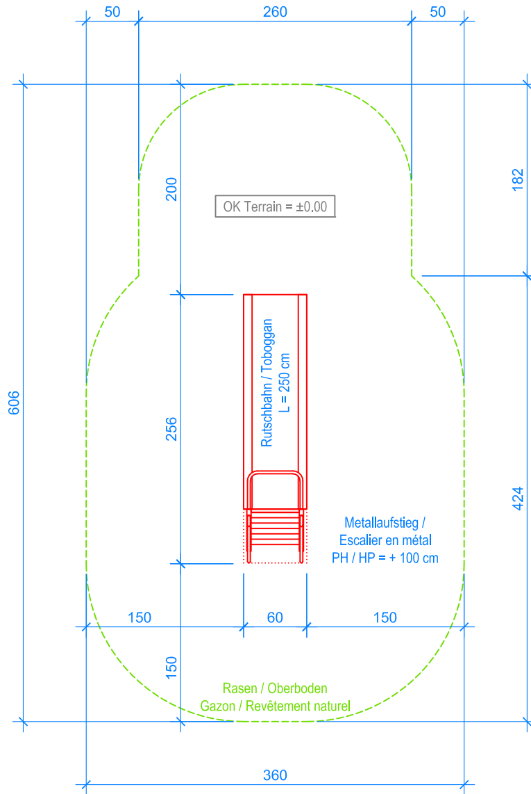
GRUNDRISS / PLAN 1:50
