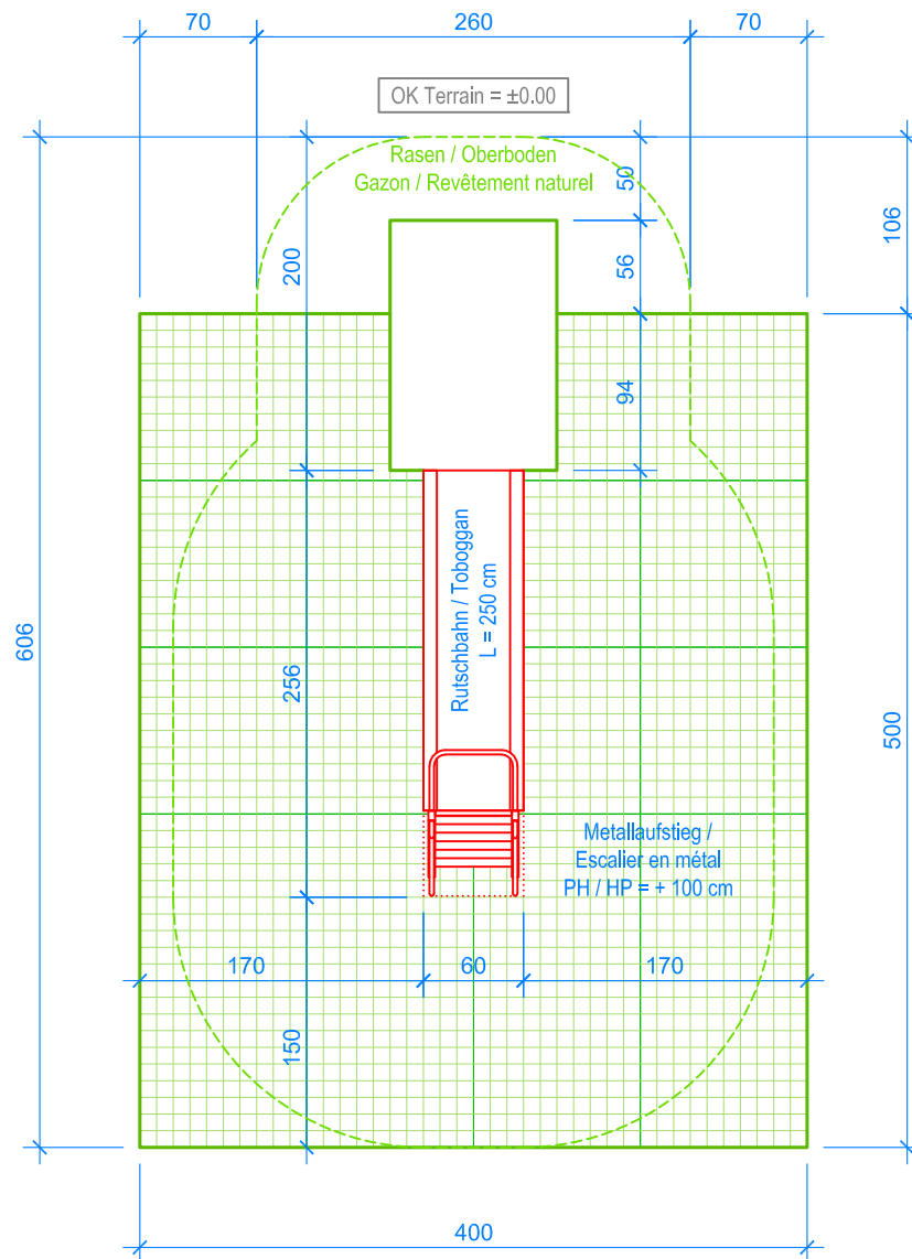
GRUNDRISS / PLAN 1:50
