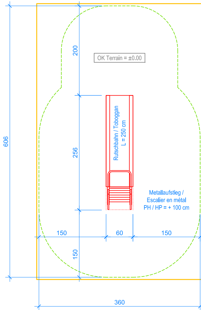
GRUNDRISS / PLAN 1:50
