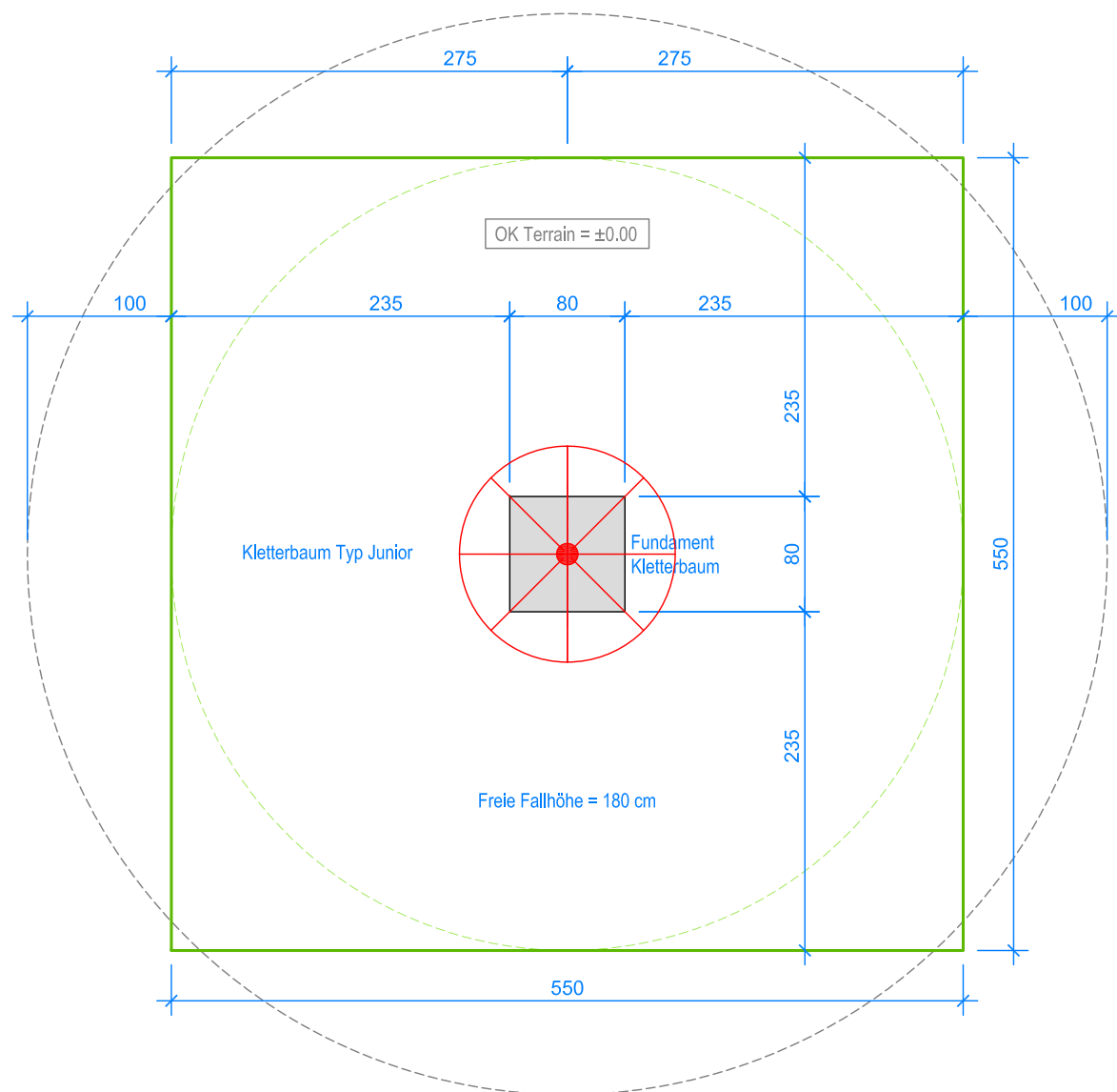
GRUNDRISS 1:50
