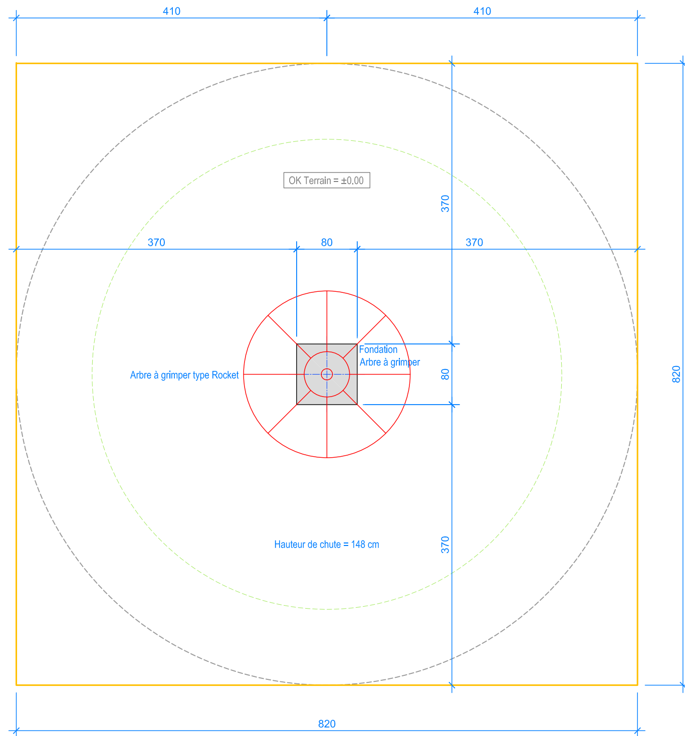
PLAN 1:50
