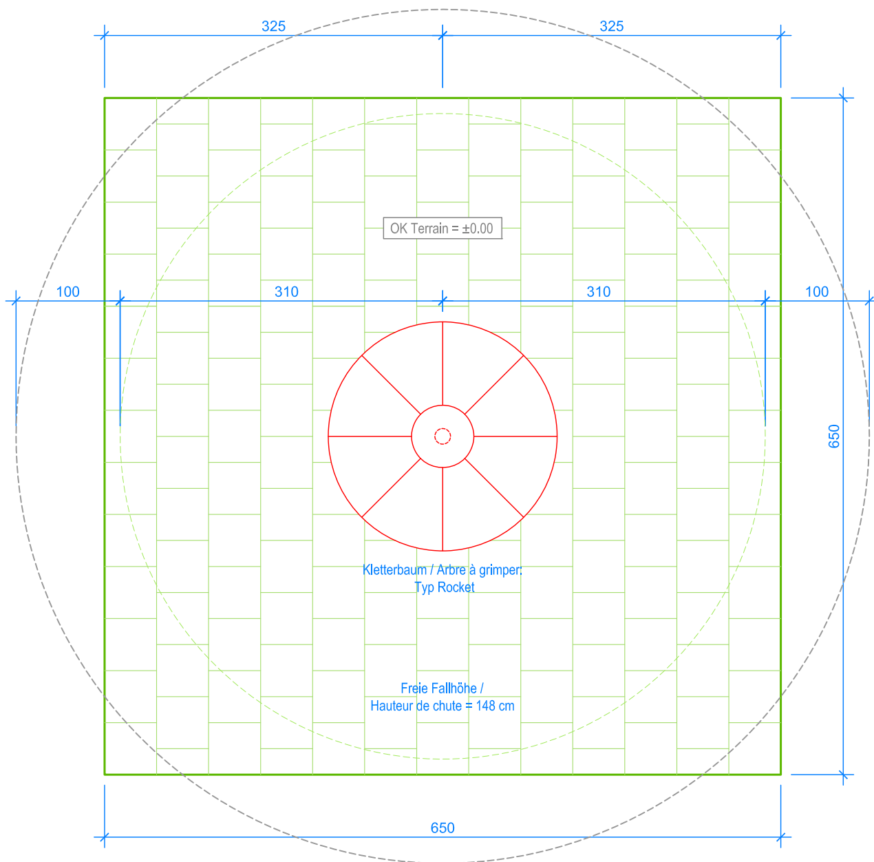
GRUNDRISS / PLAN 1:50
