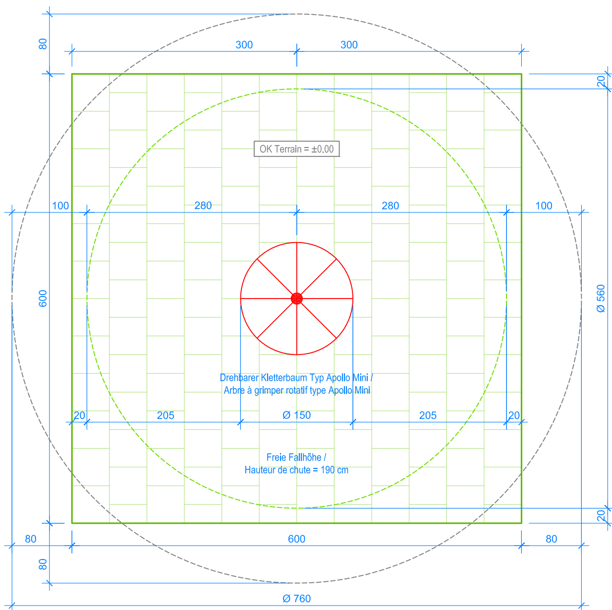
GRUNDRISS / PLAN 1:50
