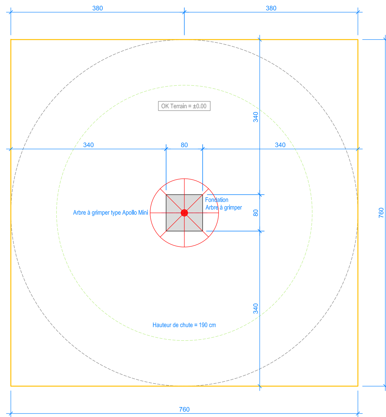
PLAN 1:50
