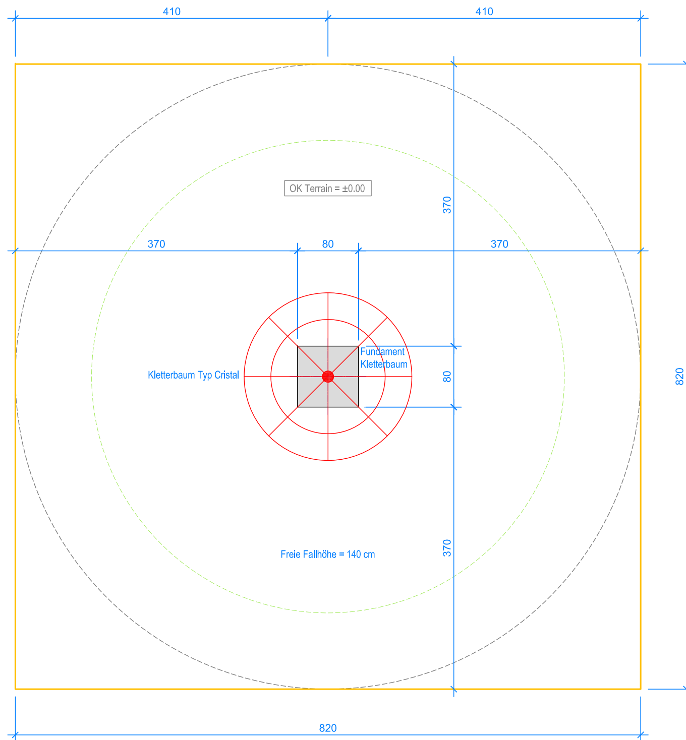
GRUNDRISS 1:50
