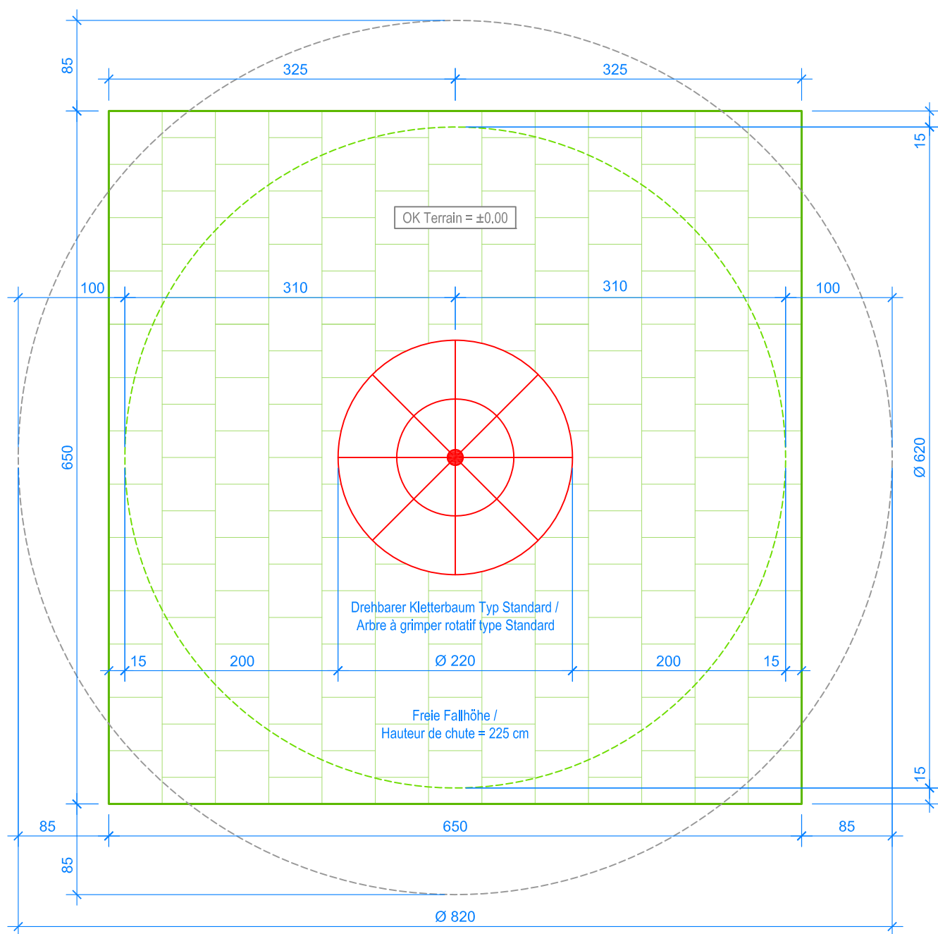
GRUNDRISS / PLAN 1:50
