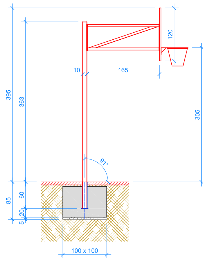
SCHNITT 1:50
