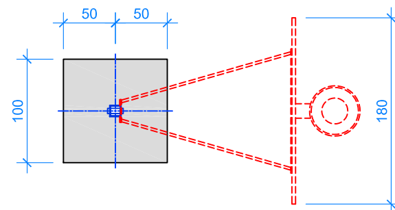
GRUNDRISS 1:50
