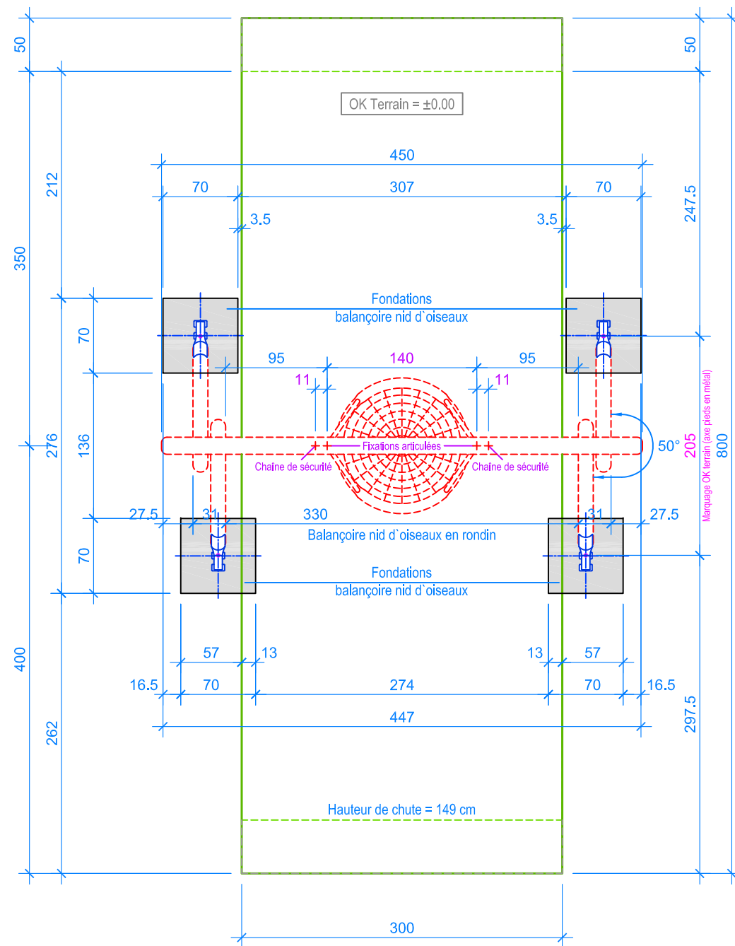
PLAN 1:50
