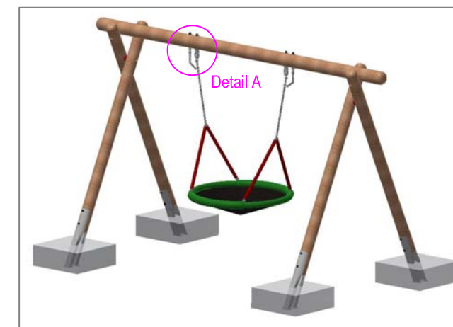
Chaîne de sécurité: Mousqueton à fixer dans le 4ème maillon
