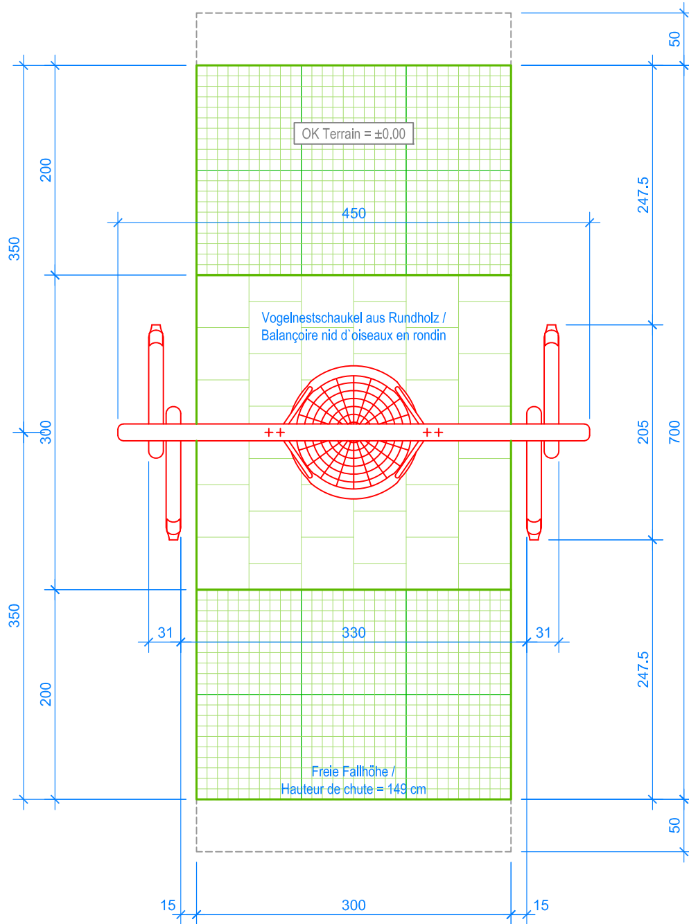
GRUNDRISS / PLAN 1:50
