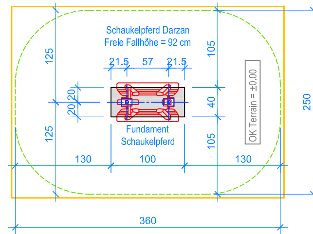
GRUNDRISS 1:50
