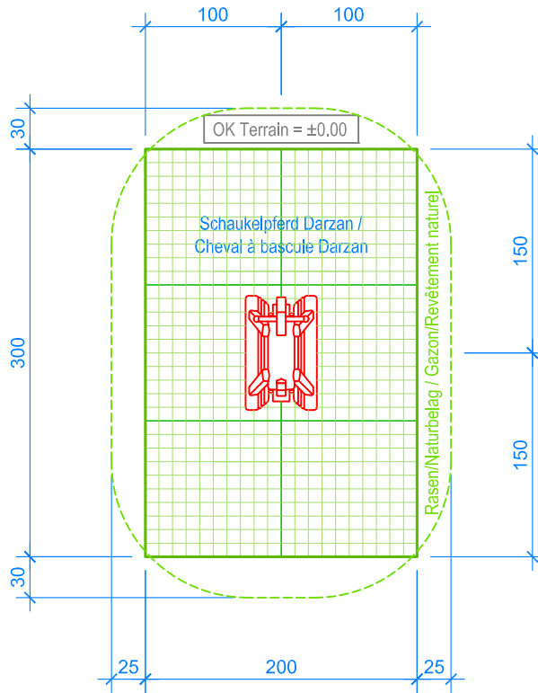
GRUNDRISS / PLAN 1:50
