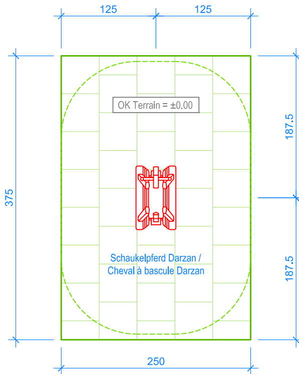
GRUNDRISS / PLAN 1:50
