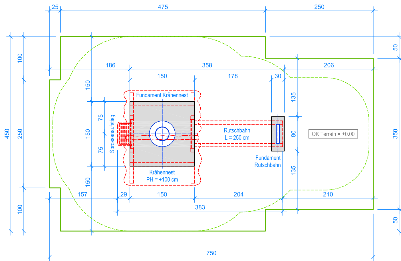
GRUNDRISS 1:50
