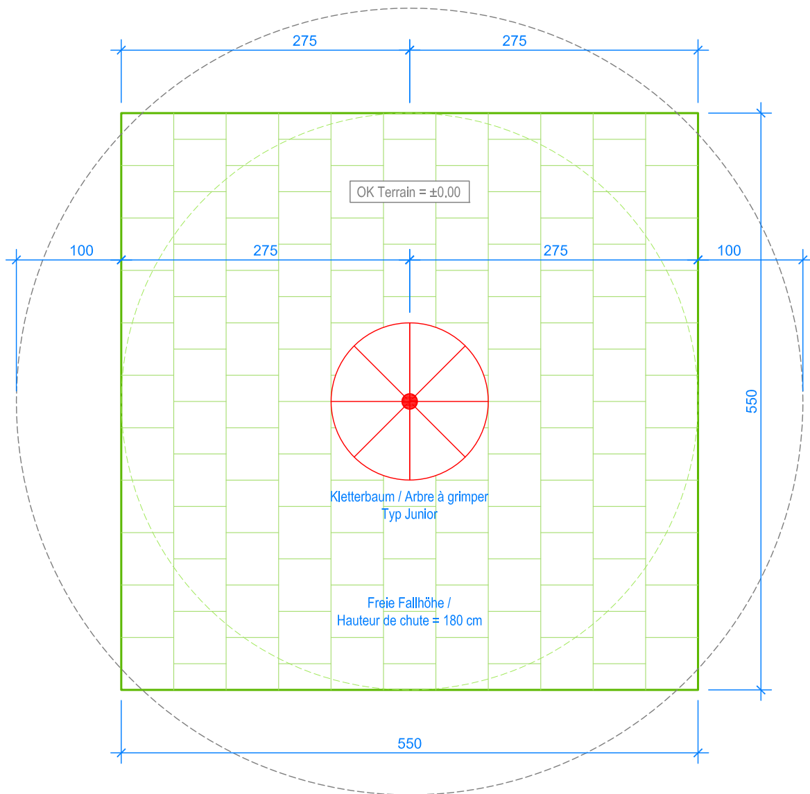
GRUNDRISS / PLAN 1:50
