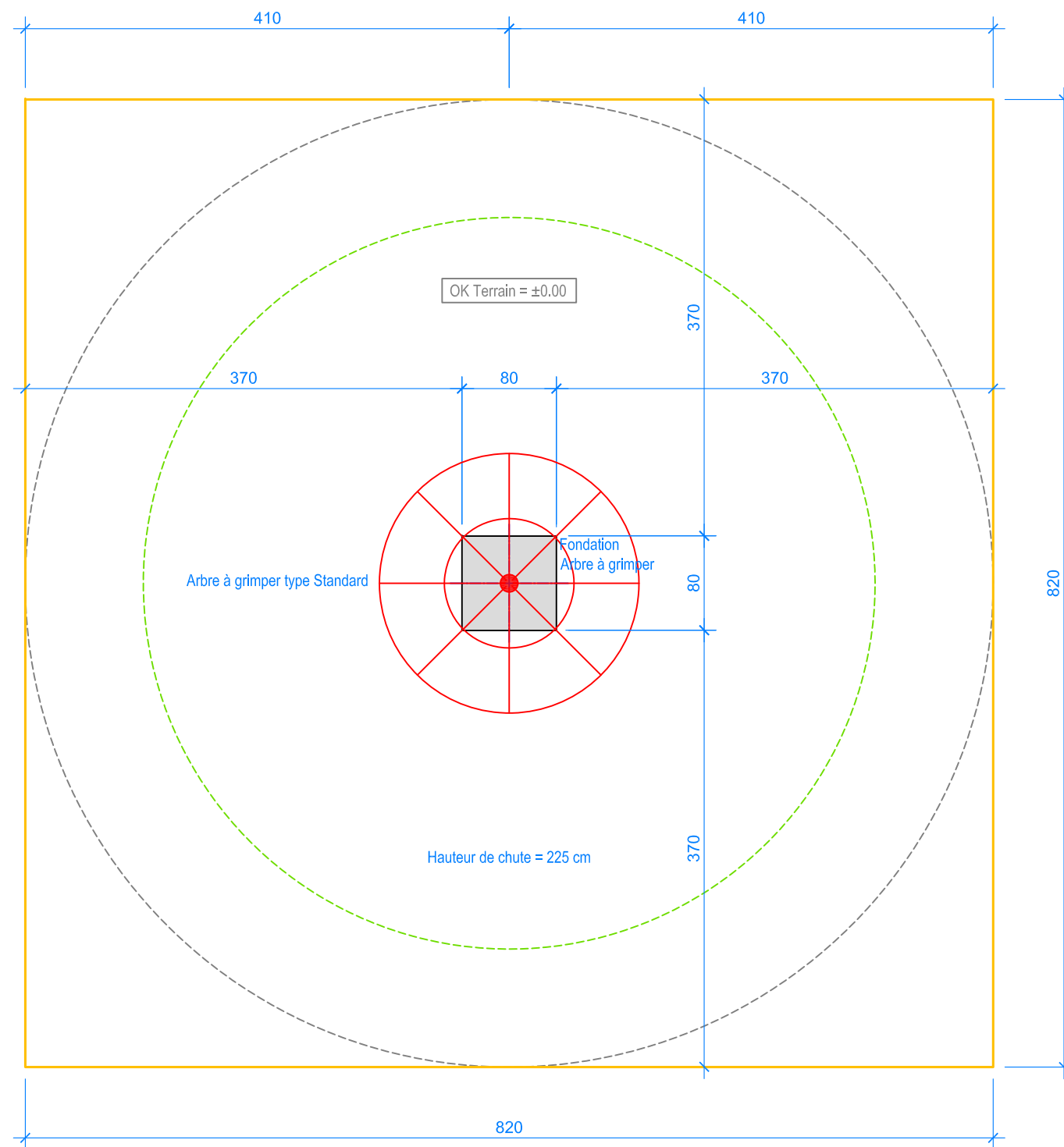
PLAN 1:50
