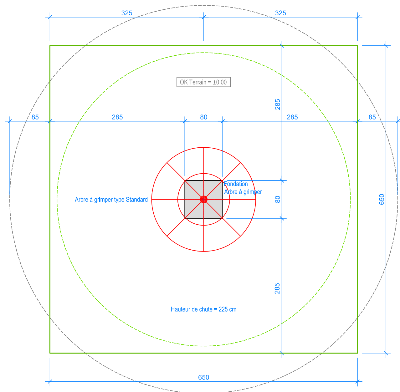
PLAN 1:50
